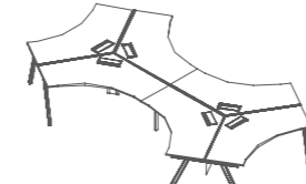
DN66 W4716*D2710*H750(mm)
