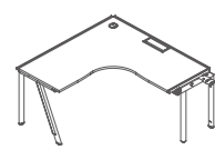
DN62AL/R W1428*D1428*H750(mm) W1528*D1528*H750(mm) W1628*D1628*H750(mm)
