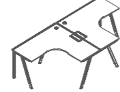
DN63 W1428*D2828*H750(mm) W1528*D3028*H750(mm) W1628*D3228*H750(mm)
