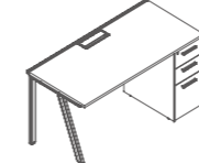
DN60 W1200*D628*H750(mm) W1400*D728*H750(mm) W1500*D728*H750(mm) W1600*D728*H750(mm)
