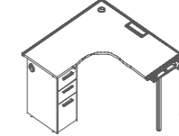
DN62BL/R W1456*D1428*H750(mm) W1556*D1528*H750(mm) W1656*D1628*H750(mm)
