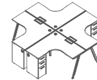
DN64 W2828*D2828*H750(mm) W3028*D3028*H750(mm) W3228*D3228*H750(mm)
