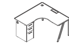
DN62L/R W1428*D1428*H750(mm) W1528*D1528*H750(mm) W1628*D1628*H750(mm)
